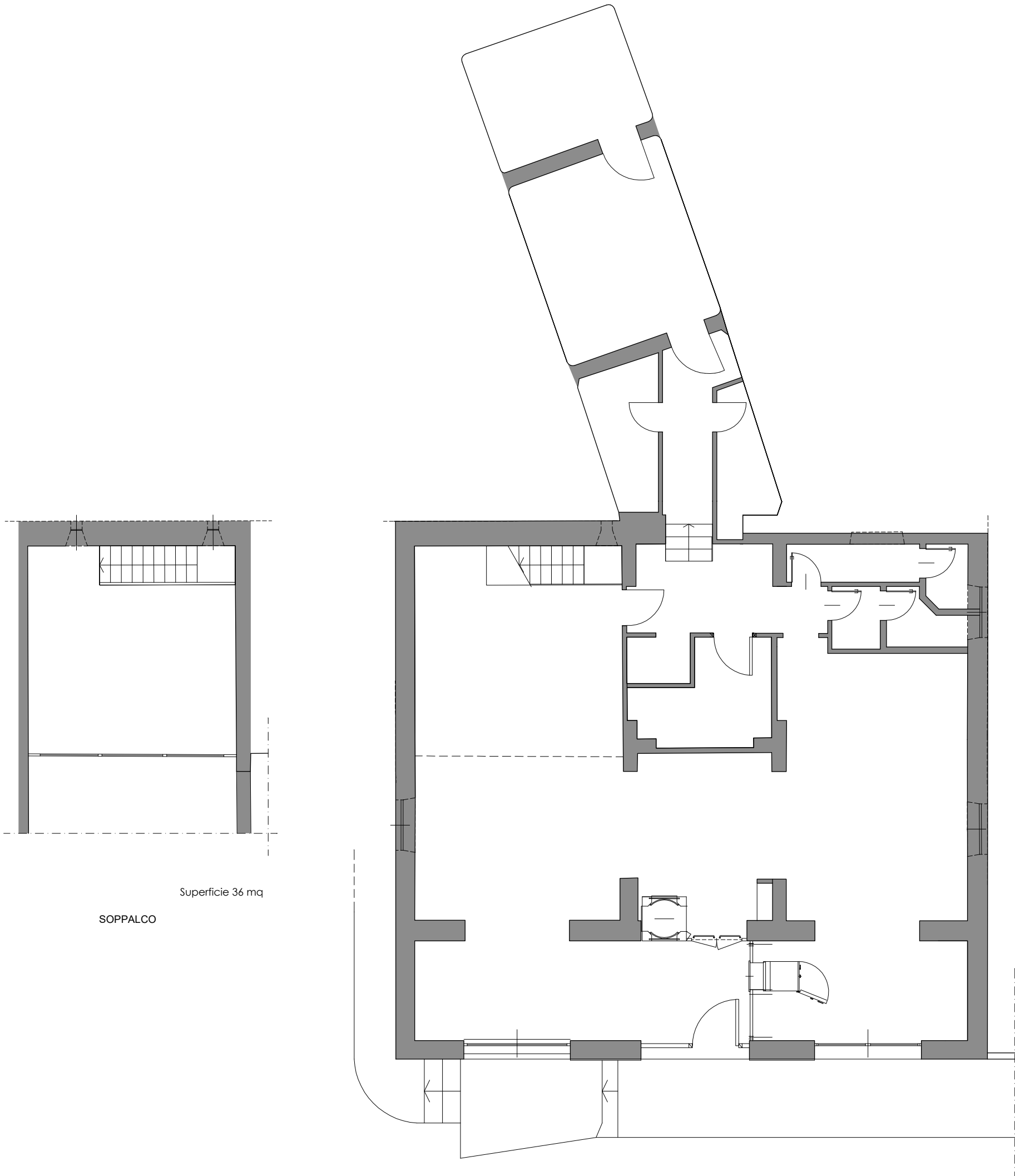
Superficie 232 mq PIANO TERRENO
